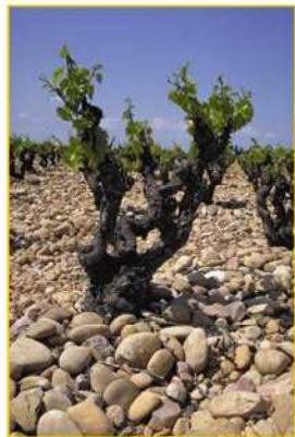
Galets du Rhône et de la Durance
